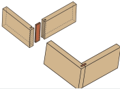
स्पलाईन जोड़
